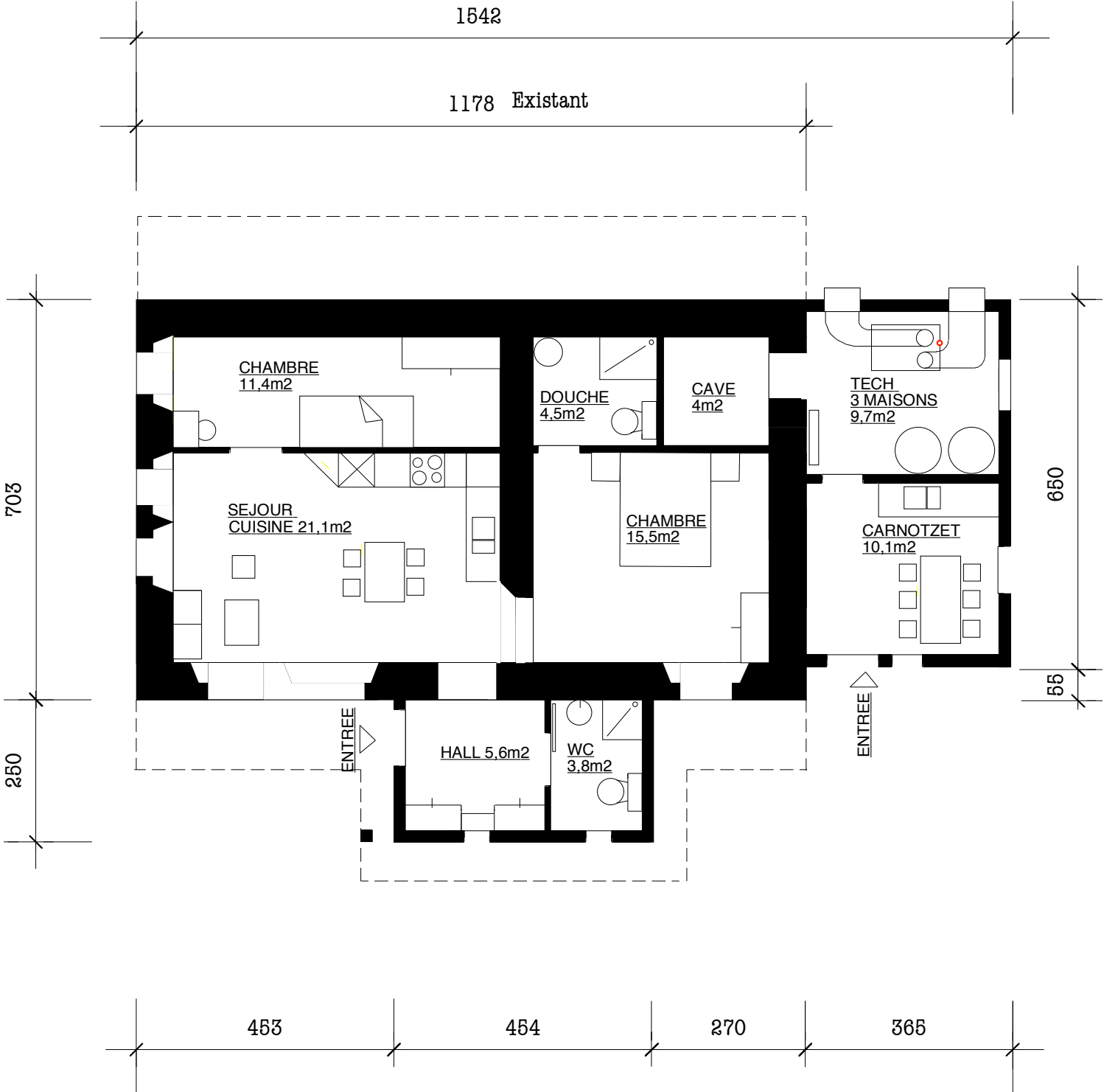
PLAN DU REZ 1/100
