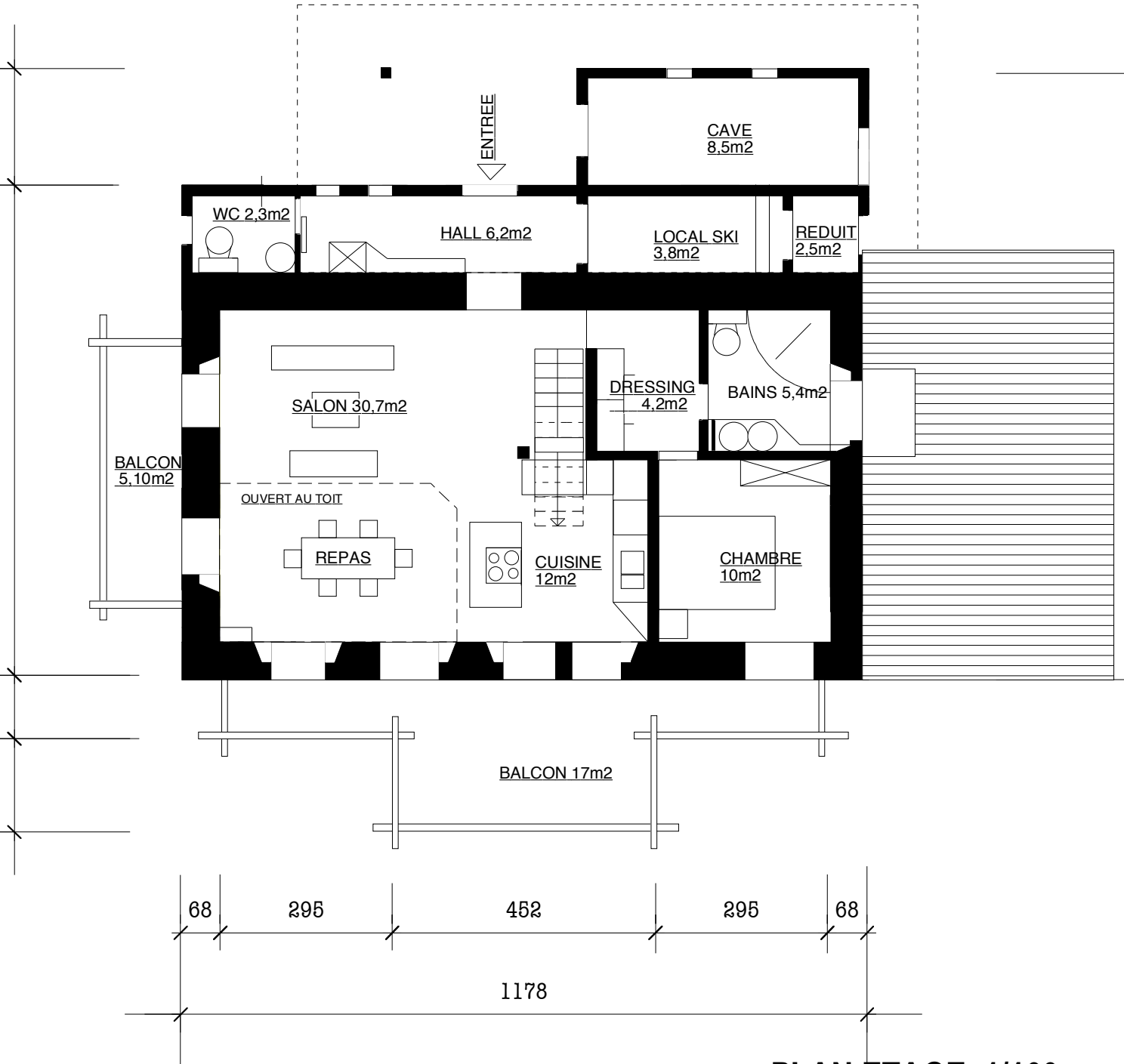
PLAN ETAGE 1/100
